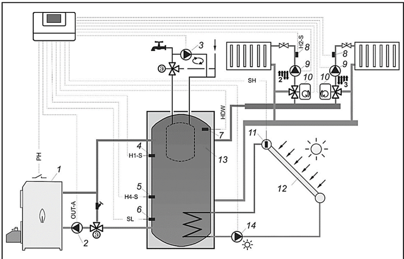
Schéma hydraulique no. 5 - diagramme avec une chaudière pellet et avec un ballon tampon 5 :
