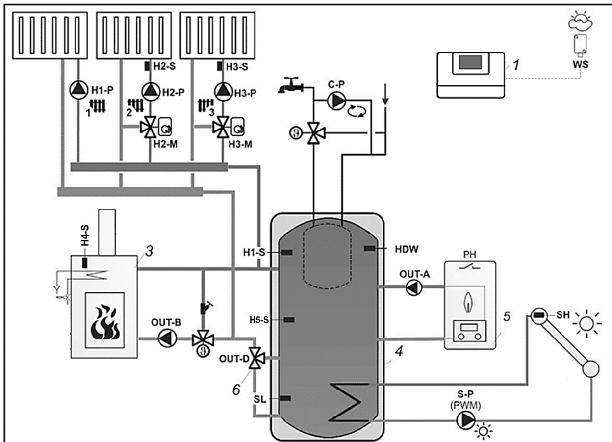
Schéma hydraulique no. 7 - diagramme "A" avec ballon tampon avec chargement du tampon par couches 7 :
