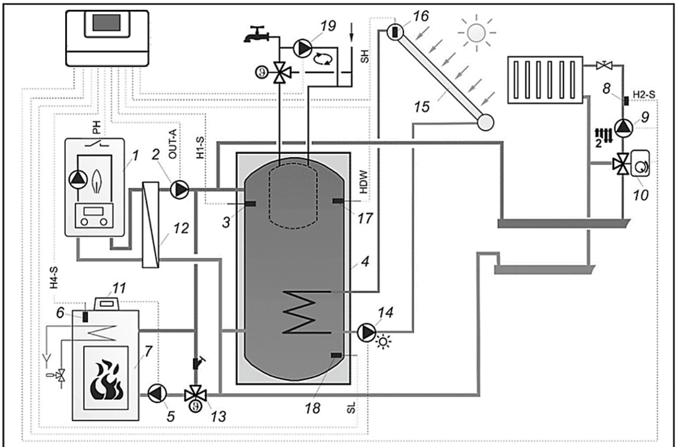
Schéma hydraulique no. 3 - Schéma avec un ballon d'ECS en bain-marie et solaire 3 :
