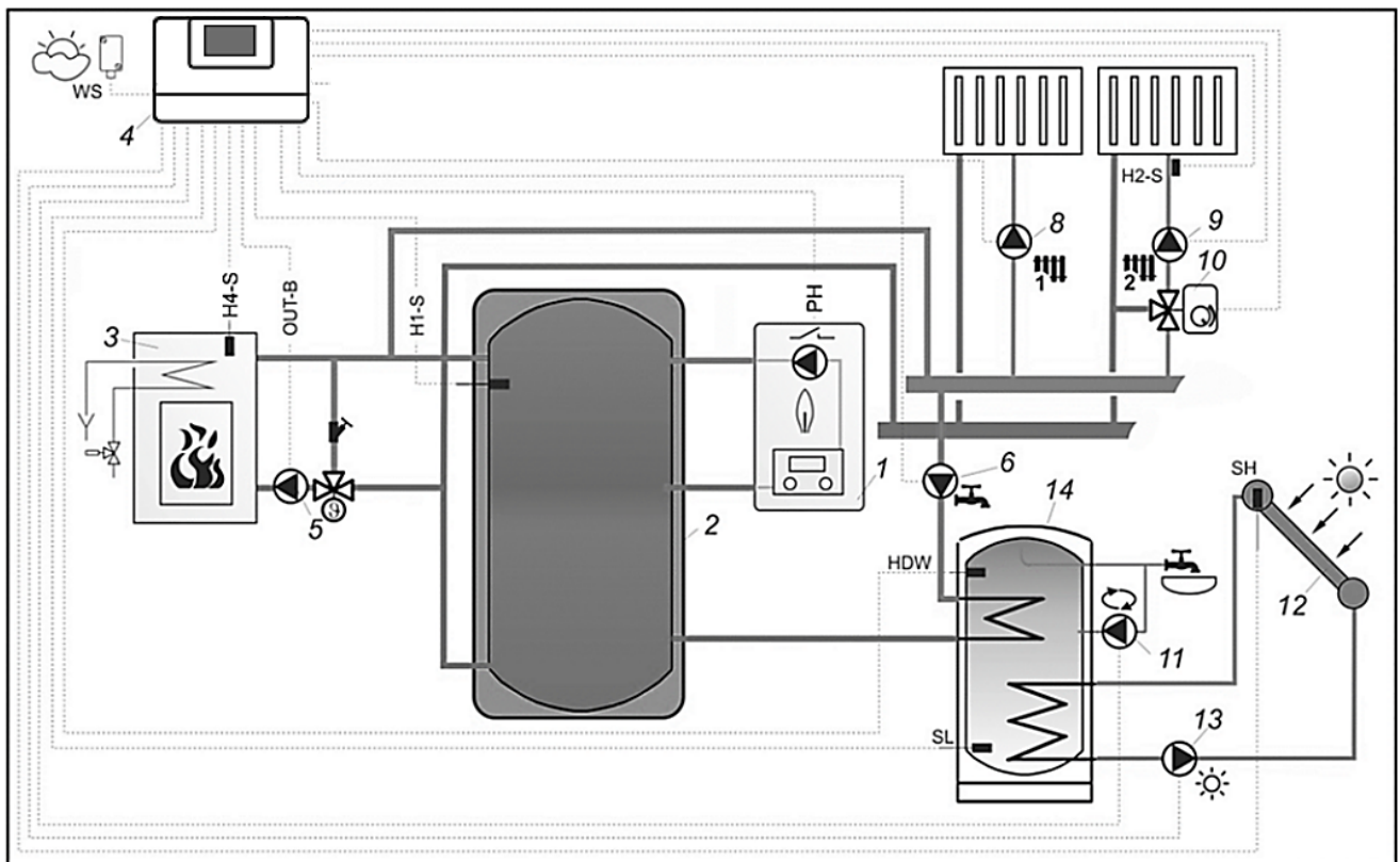
Schéma hydraulique no. 8 – diagramme "B" avec ballon tampon avec chargement du ballon tampon par couches 8 :
