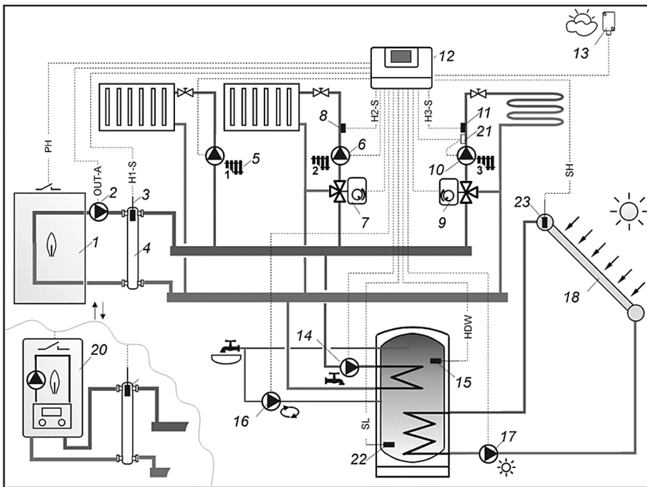
Schéma hydraulique no. 1 – schéma de base 1 :
