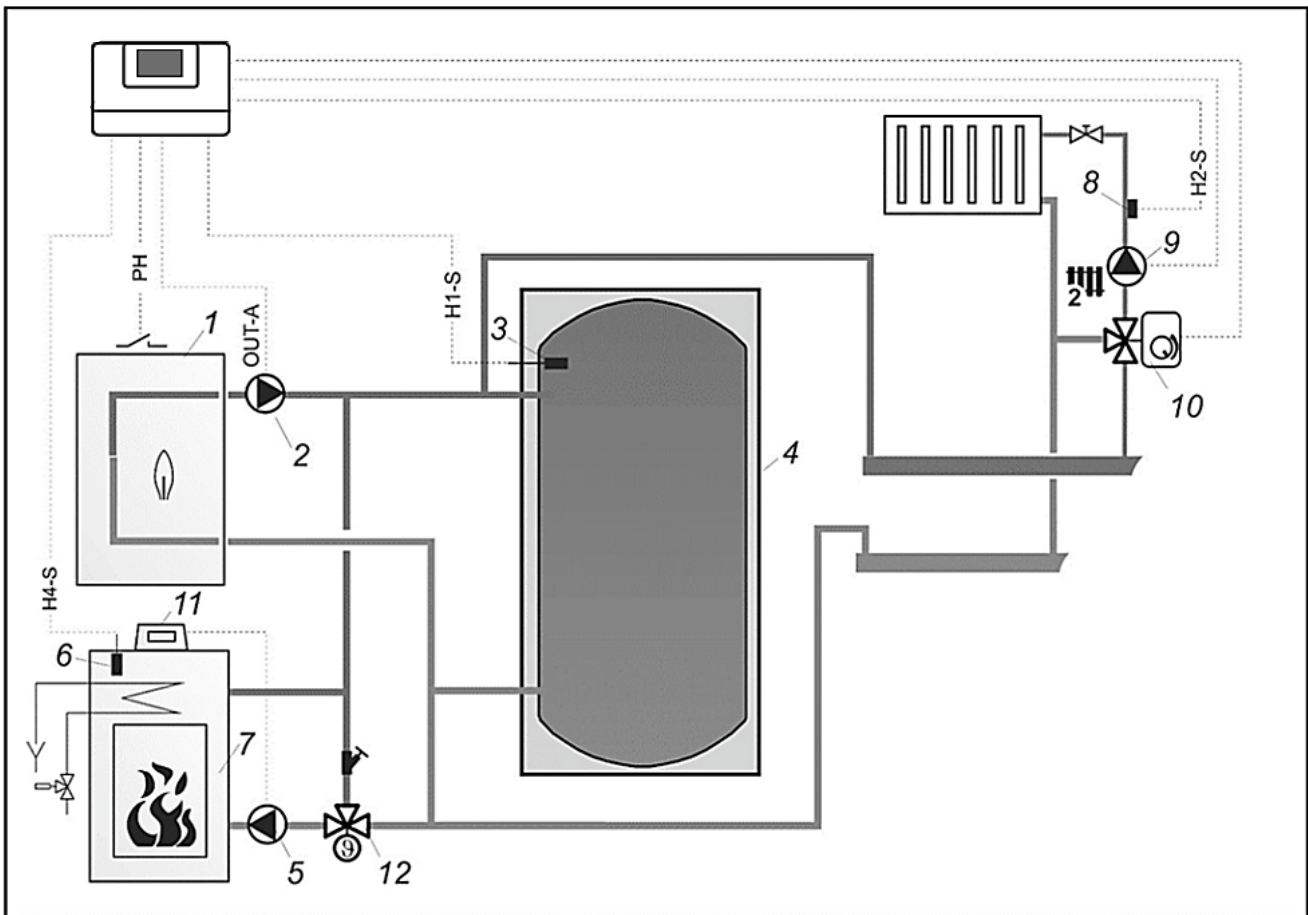
Schéma hydraulique no. 4 - diagramme "B" avec ballon tampon 4 :
