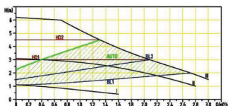
11.5. SALUS MP200/MP280A Curba de performanță
