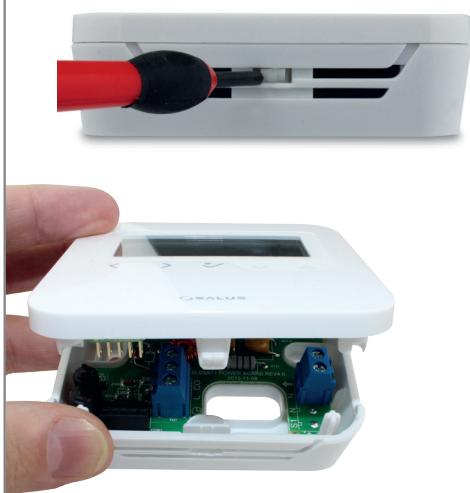
Demontage des Gehäuses von der Grundplatte
