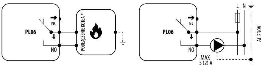
Schemat podłączenia pompy i kotła z modułem (dla KL06)
