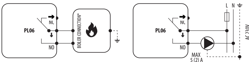
Anschlussplan des Pumpen- und Brennerlogikmoduls (für KL06)
