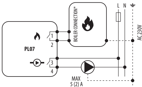
Anschlussplan des Pumpenlogikmoduls (für KL06)
